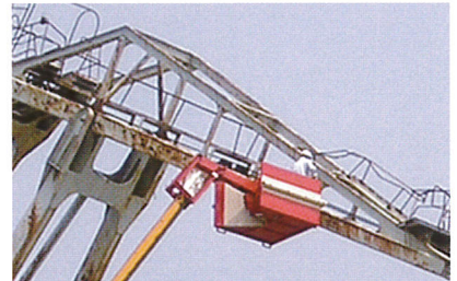
避雷針交換作業 半径30m 50Tラフター
